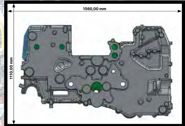
| Wasserführgehäuse in den Abmessungen des Formkastens
