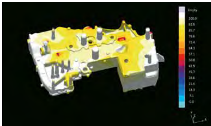
Erstarrungssimulation
