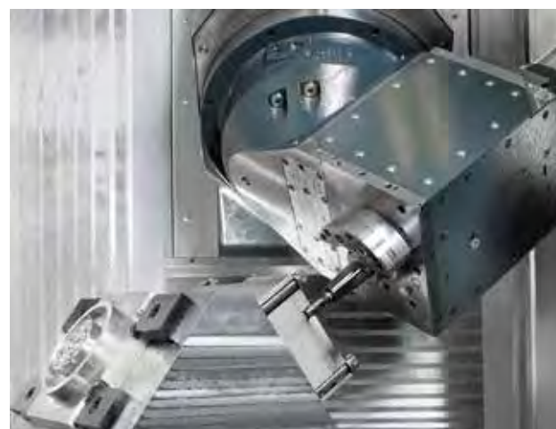
| Detailansicht Fräbkopf der 5-Achs-Maschine
